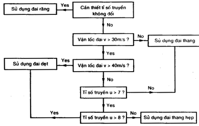
Hình 4.30 Sơ đồ chọn loại đai
